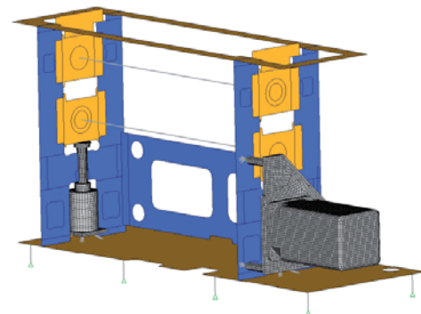
Verarbeitungsmaschinen
